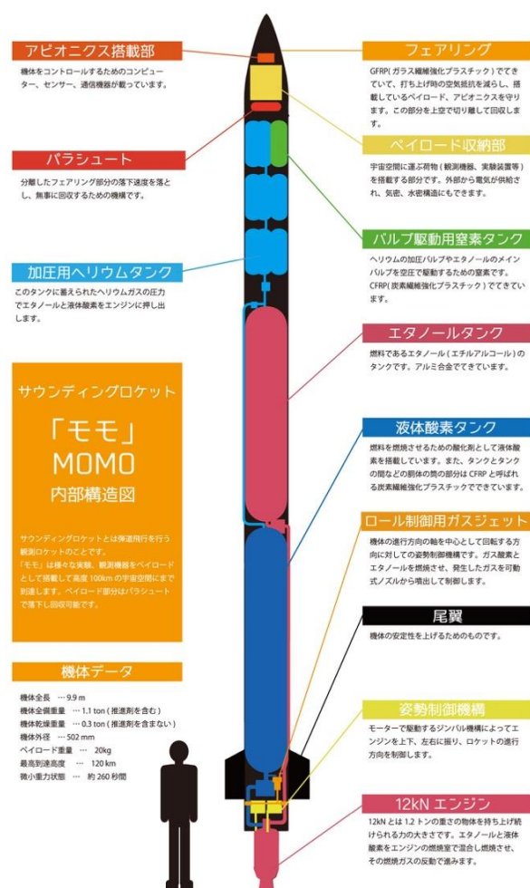
図 2: サウンディングロケット「モモ」MOMO 内部構造図 ( http://www.istellartech.com/technology/momo )
